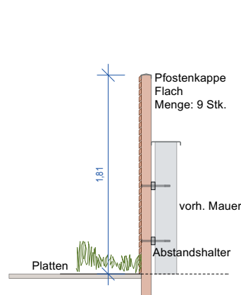
Schnitt A-A'
